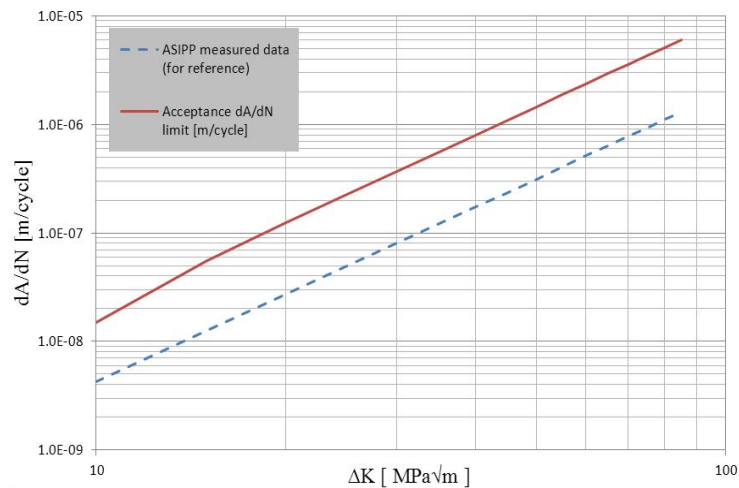
图 2. 1 FCGR 测试接收标准图
