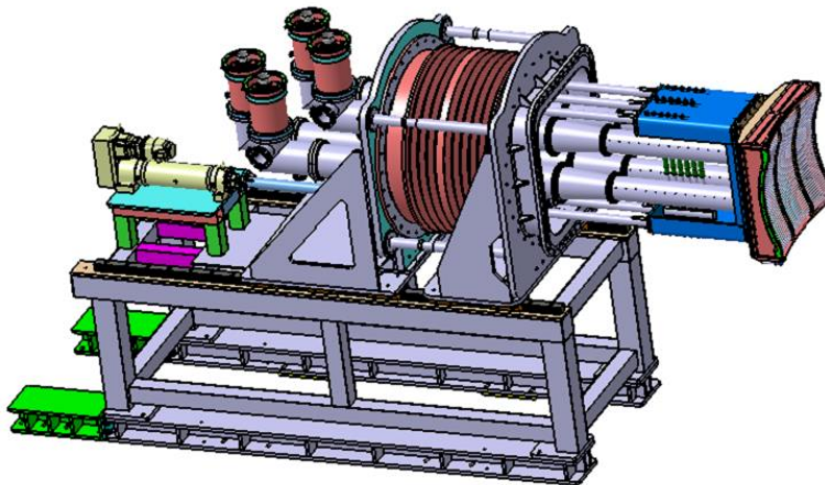
图 2 天线结构示意图
