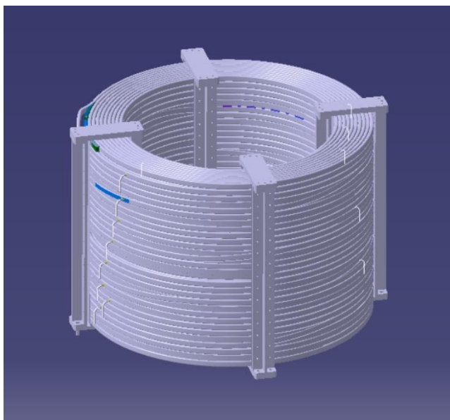
图 1 BEST CS LTS 线圈绕组
