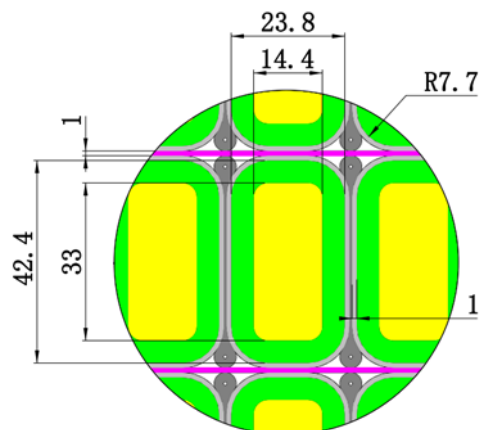
图 2 BEST CS LTS 导体
