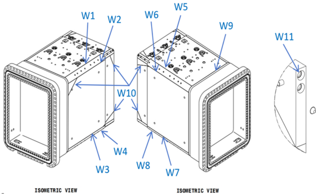
图2 水平窗口插件电子束焊缝
