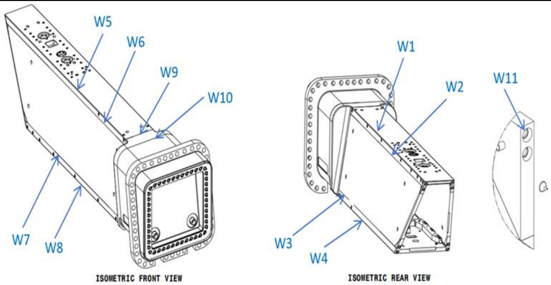
图 1 上窗口插件电子束焊缝
