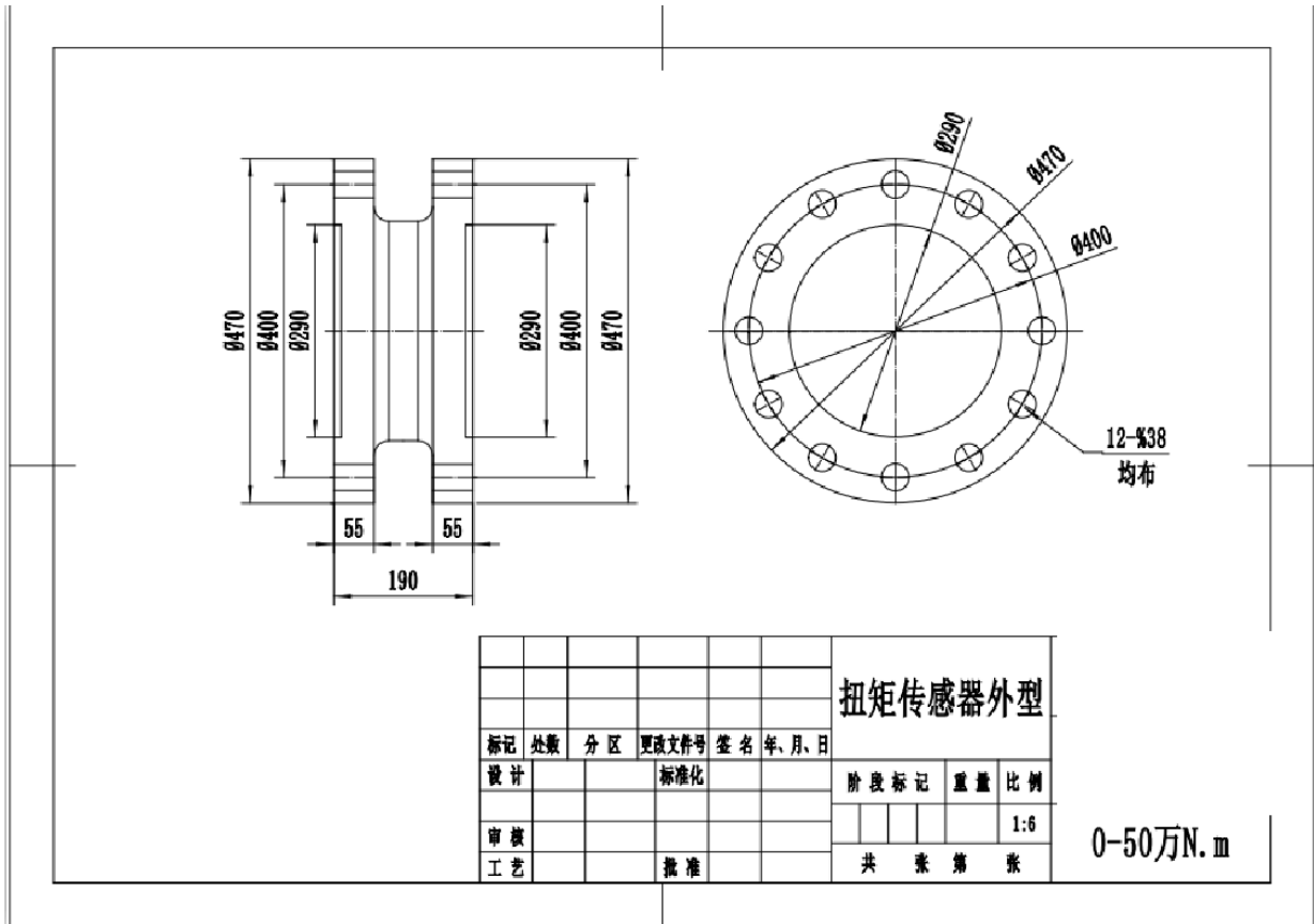
500000N.m 扭矩传感器外形尺寸图纸
