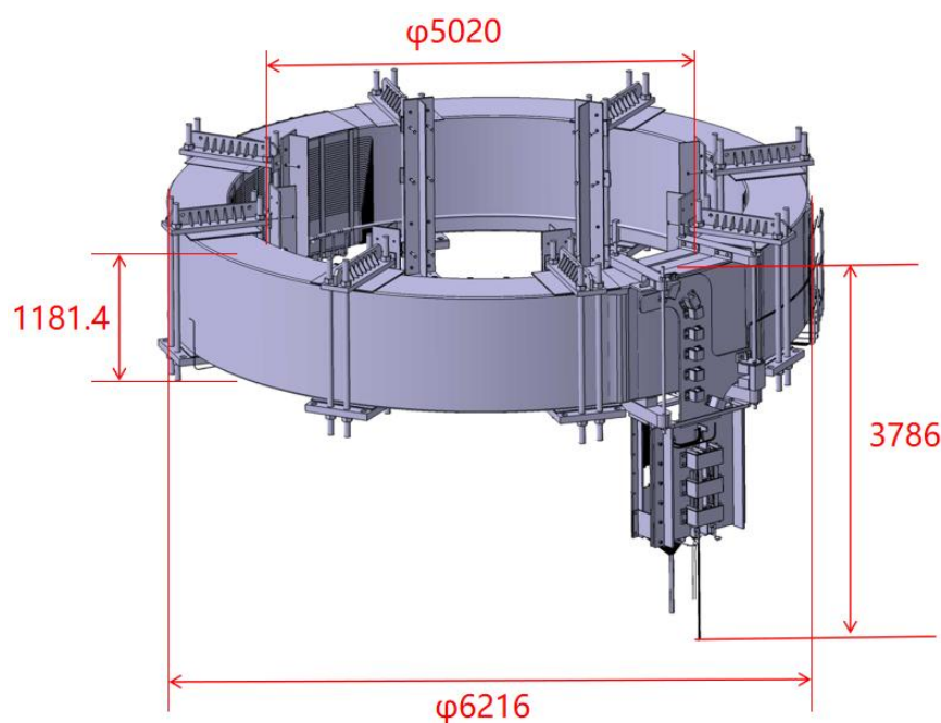
图 PF6 磁体结构尺寸及模型
