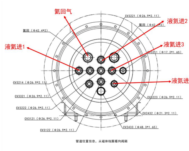
图2 内部低温管道和原阀箱管道对接信息
