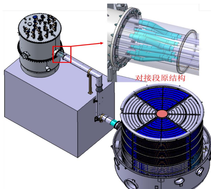
图1 CSMC测试阀箱示意
