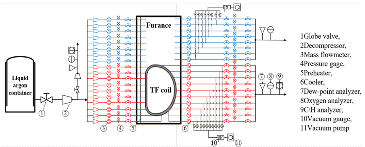
图：磁体热处理氩气保护系统示意图
