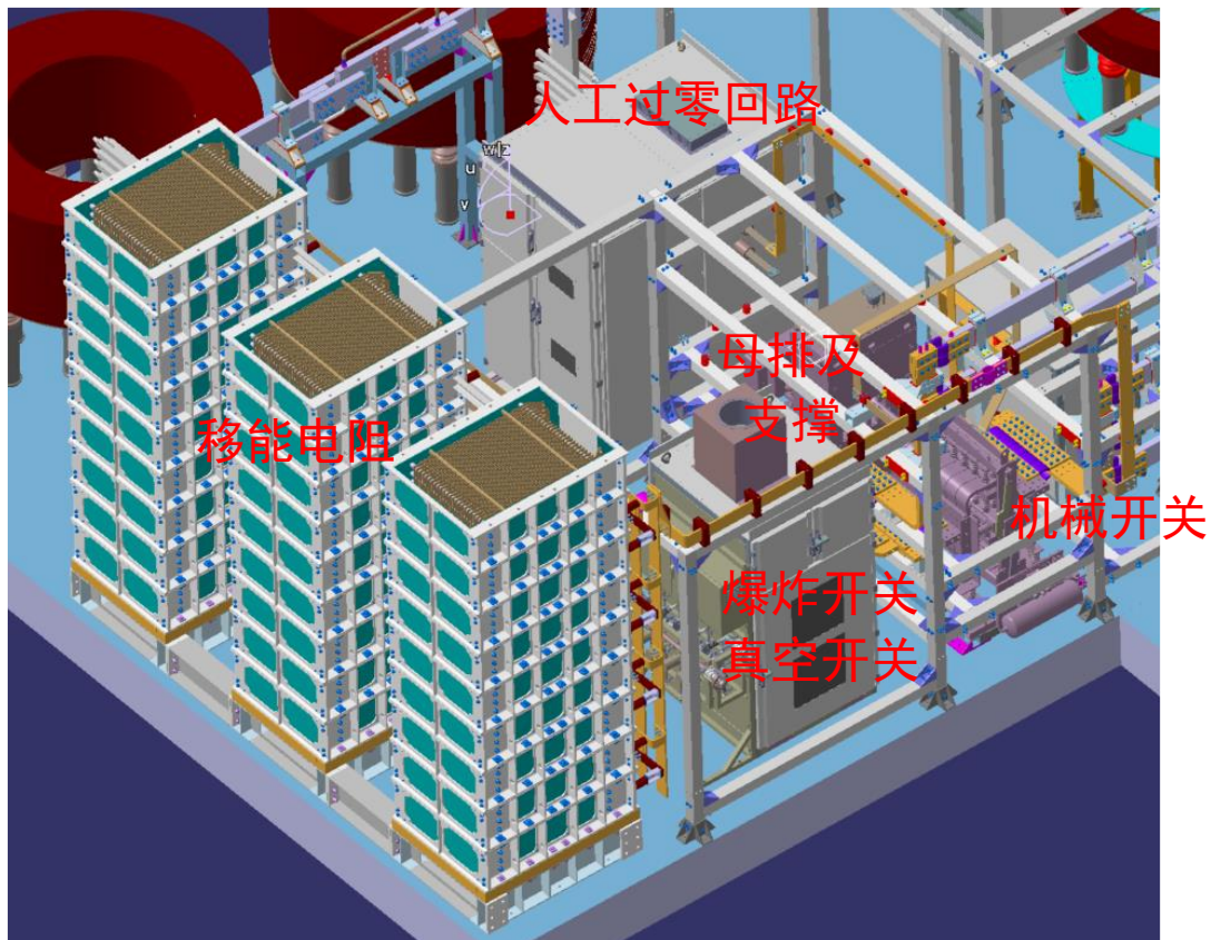
图 2：布局图
